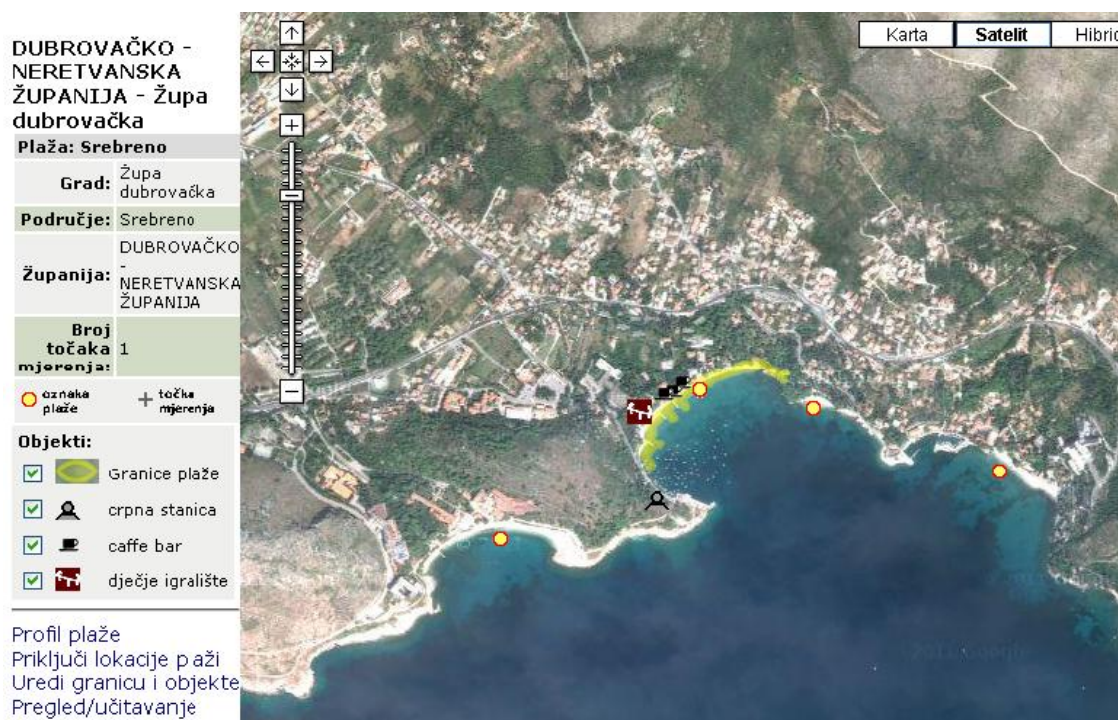
Slika 5. Profil plaže Srebreno u Župskom zaljevu.
